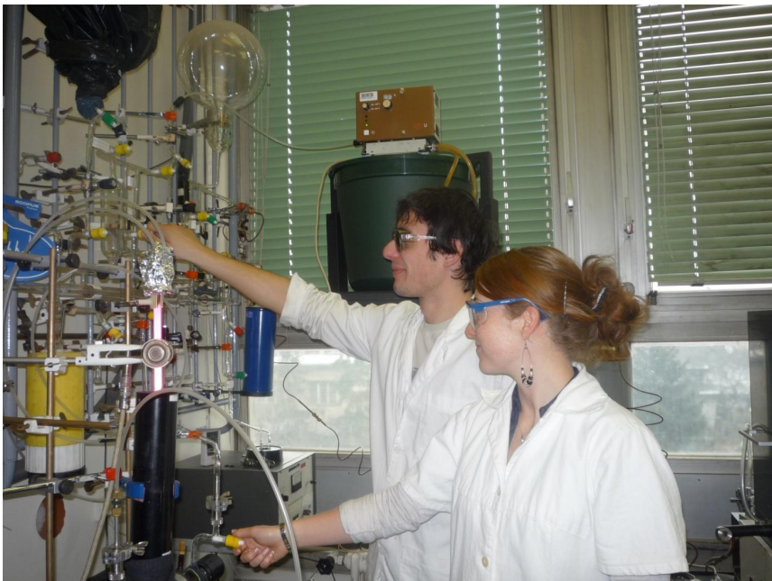
Az OH-gyök detektálására használt rezonancia-fluoreszcencia mérővonal beállítása reakciókinetikai mérésekhez
